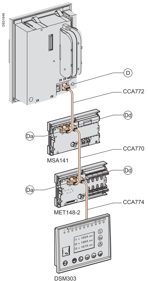
Пример подключения выносных модулей к Seram серии 20
