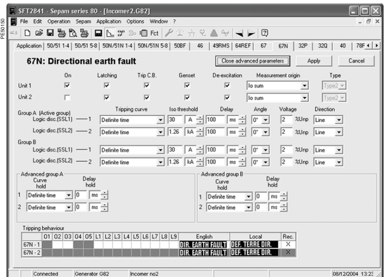
Окно настройки направленной защиты от замыкания на землю
