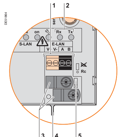
Порт E-LAN (ACE969TP или ACE969FO)
